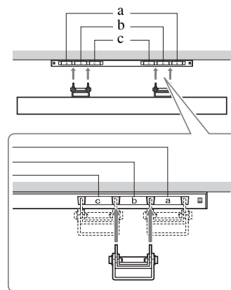
Umístění závěsů
