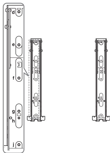
Umístění šroubů
