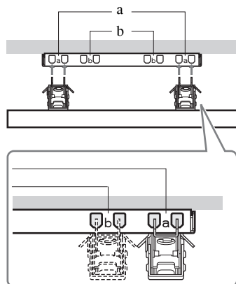
Θέση άγκιστρου
