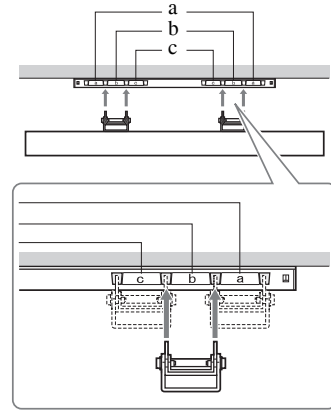
Kanca yeri
