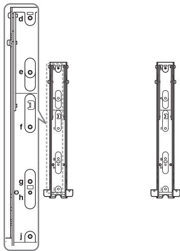
Skruvarnas placering
