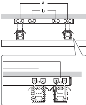
Kanca yeri
