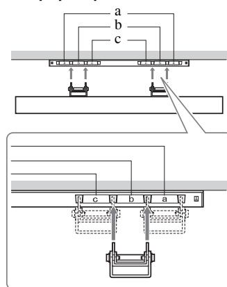
Θέση άγκιστρου
